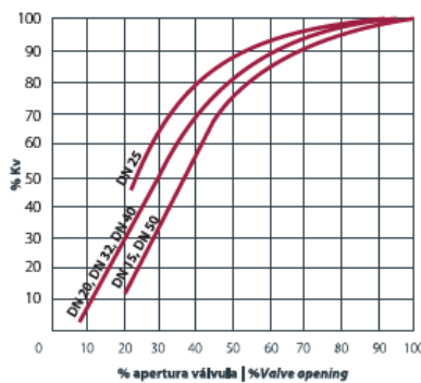
Flujo relativo Relative flow
