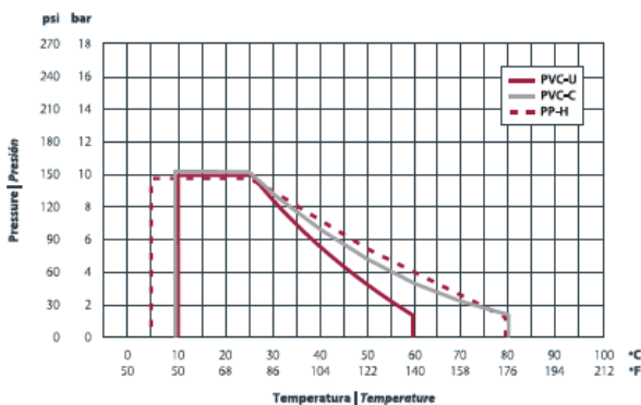
Presión vs. temperatura Pressure vs. temperature
