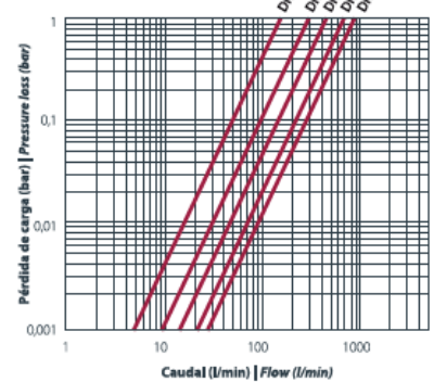
Pérdida de presión Pressure loss
